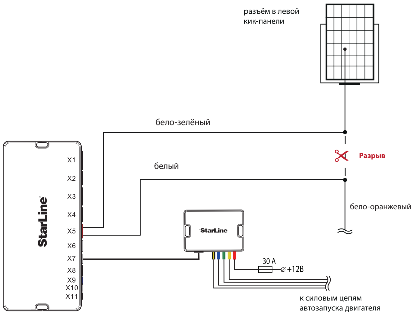
Схема 1. Подключение цепей автозапуска двигателя и обхода штатного иммобилайзера
