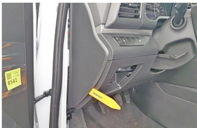
Фото 1.7. Снять боковую накладку передней панели
