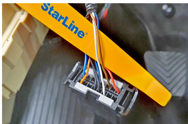
Фото 3.5. Шина CAN-B (белый и коричневый)
