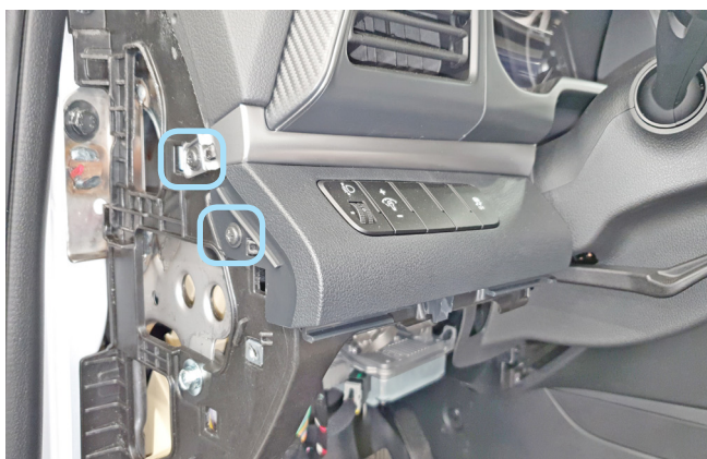
Фото 1.11. Саморезы крепления декоративной накладки и блока кнопок
