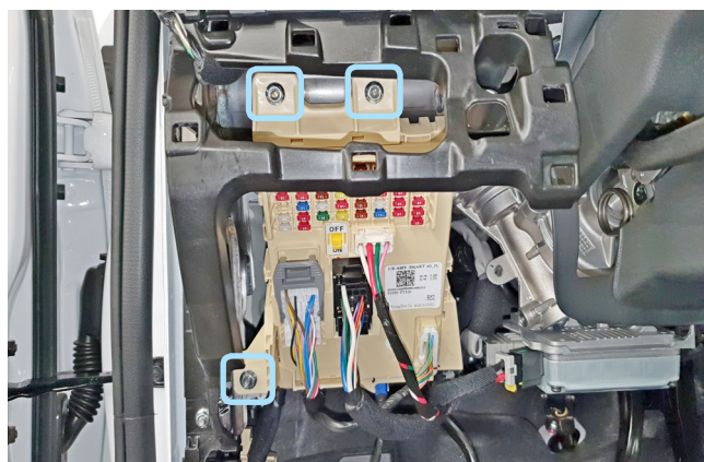
Фото 1.14. Крепление монтажного блока предохранителей
