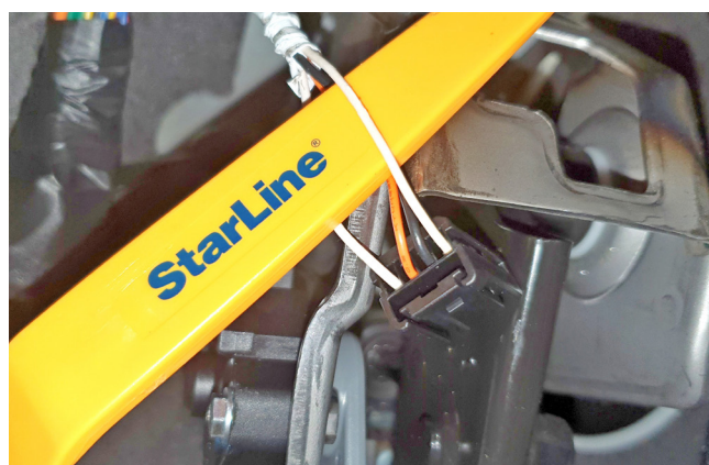
Фото 3.14. Стартер (белый)
