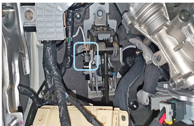
Фото 3.8. Местоположение разъёма
